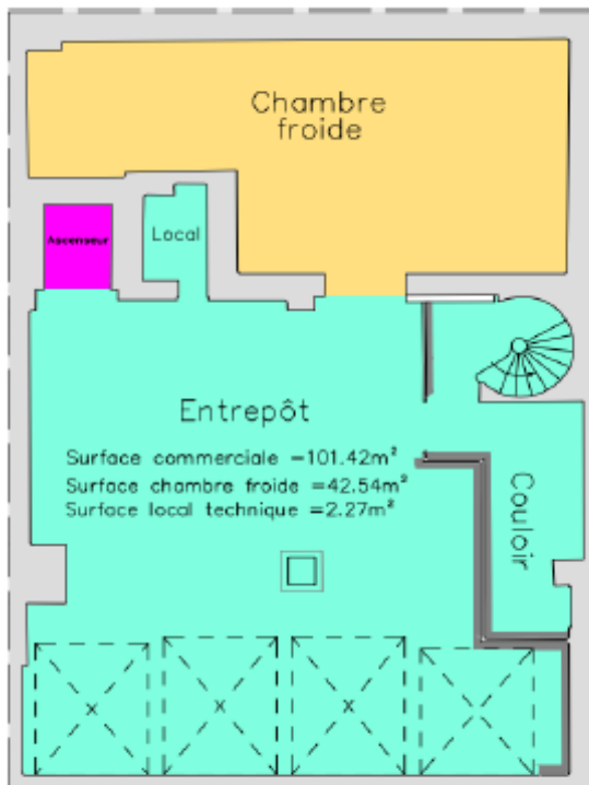
Plan figuratif du RDC - Entrepôt
